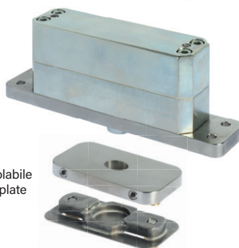
CERNIERA INFERIORE CON FERMO A MOLLA OGNI 90 GRADI E RICHIAMO DI 20° PRIMA DELLA POSIZIONE DI FERMO.
